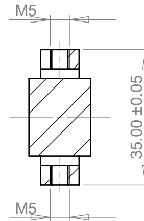
COUPE A-A
