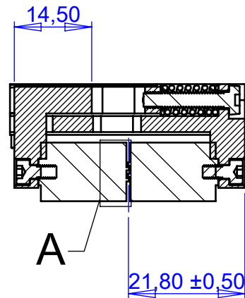
COUPE A-A
