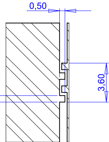
DÉTAIL A ECHELLE 5 : 1
