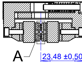
COUPE A-A
