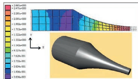
Fig. 2: Horn sonotrode FEA.
